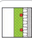
NB1 Rohrsystem auf Dämmplatte im Nassestrich *P1 / P2 / P6 / P7 / P8
