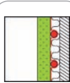
NB2 Rohrsystem in Dämmplatte mit Nassestrich *P1 / P2 / P6 / P7 / P8
