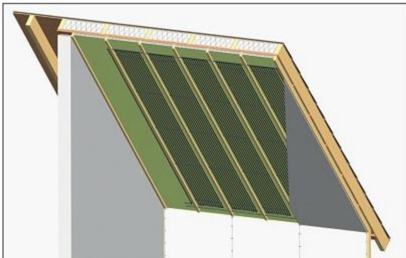
Verlegung der Rohre, Register in Dachschrägen.
