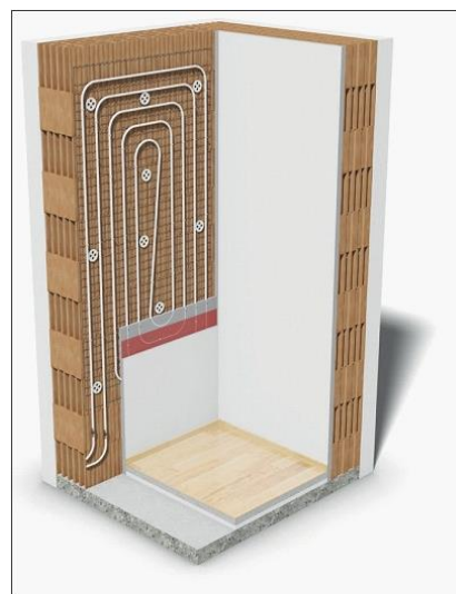
Verlegung der Rohre, Register, Heizleitungen und Flächenheizelemente direkt auf der Wand mit Wandputz.
